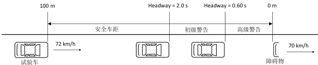
图 8-1 车距监控实验过程示意图
